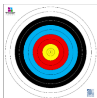
Osatua (10 – 1): 122: 122 cm Ø 80: 80 cm Ø 40: 40 cm Ø
