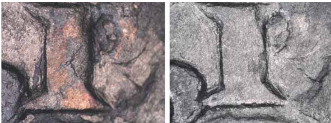
Figura 6.- Detalle de algunas de las zonas “cobreadas” antes y después de la eliminación de los depósitos.
